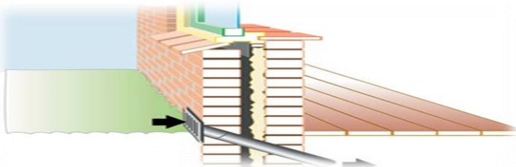
Ubbink Ondervloer ventilatierooster
